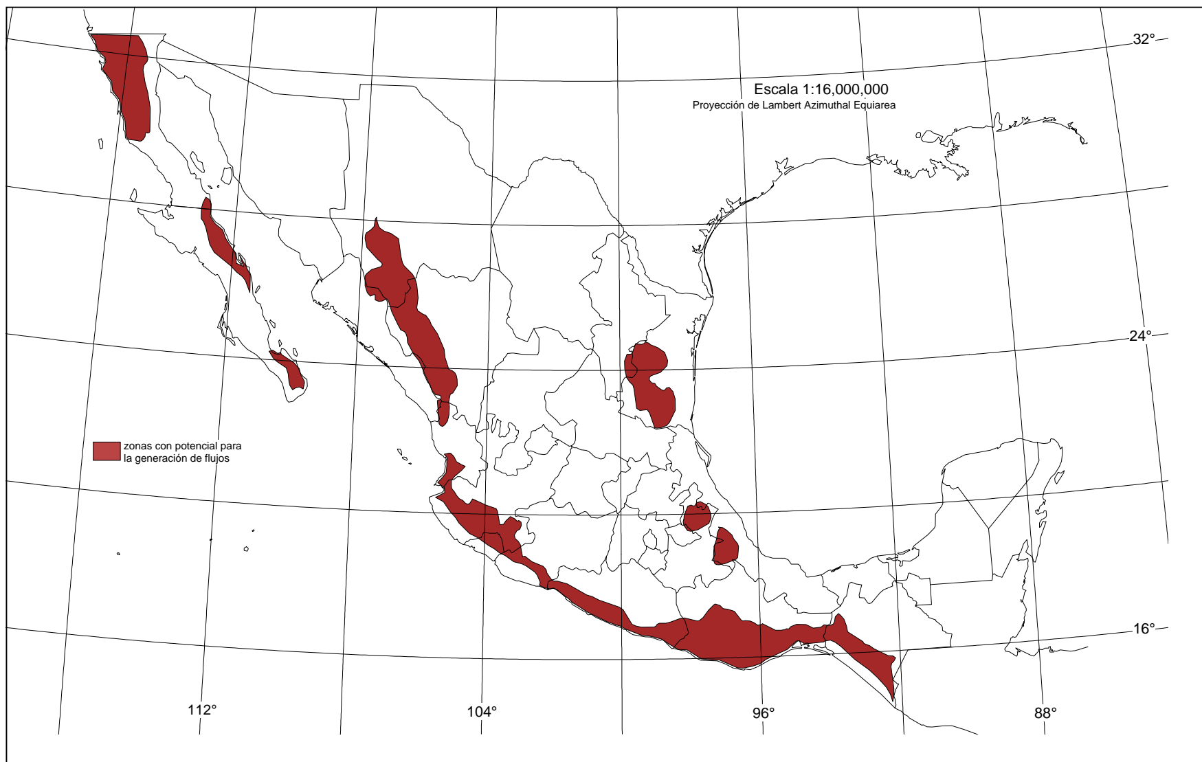
Figura 56. Flujos de lodo y escombros por lluvia
