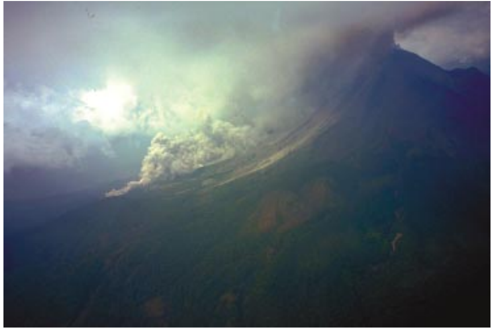
Figura 37. Flujos piroclásticos
